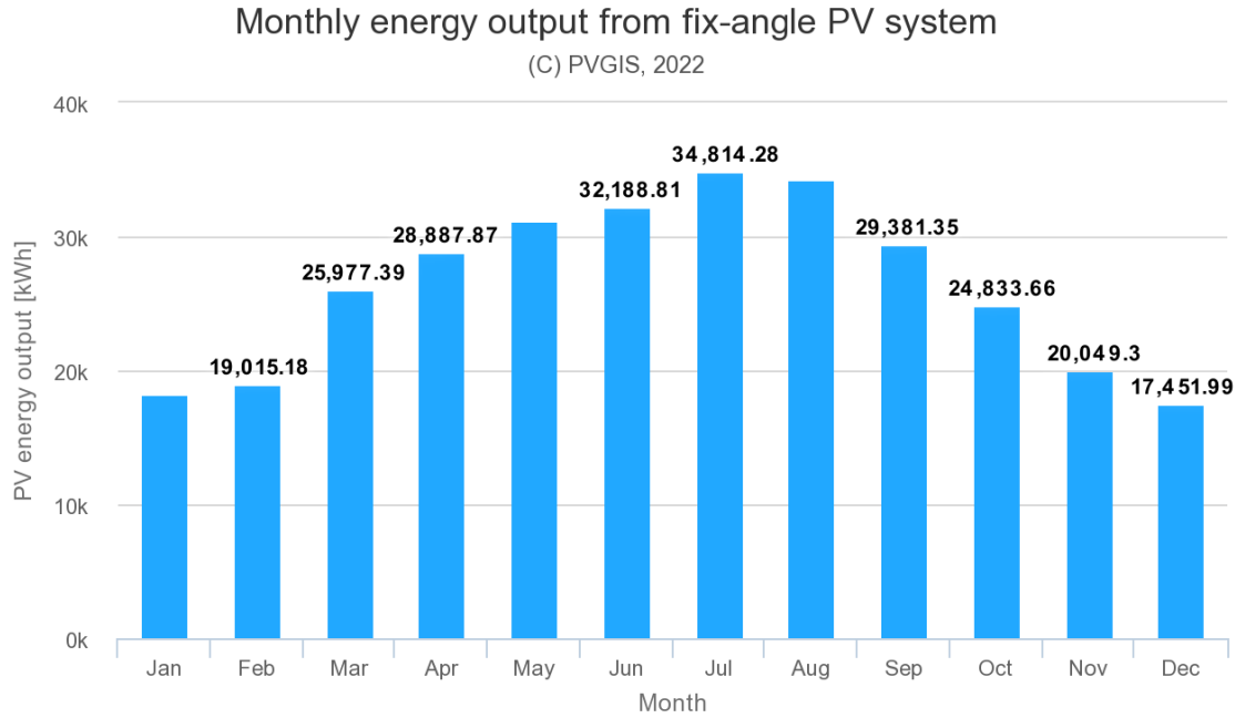
Σχήμα 2: Μηνιαία παραγωγή ηλεκτρικής ενέργειας (kWh)
